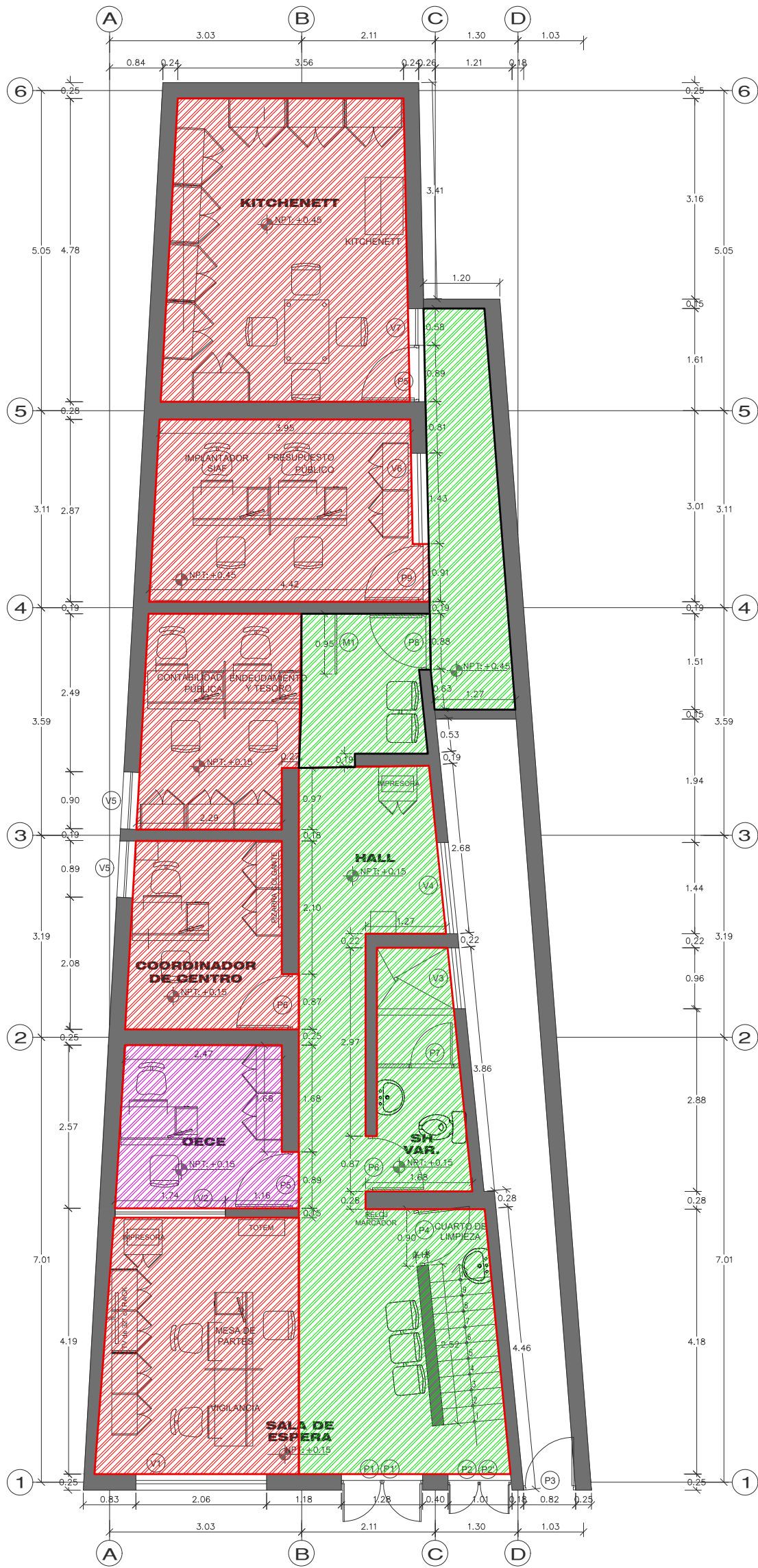
DISTRIBUCIÓN ACTUAL DE ARQUITECTURA DEL PRIMER NIVEL
