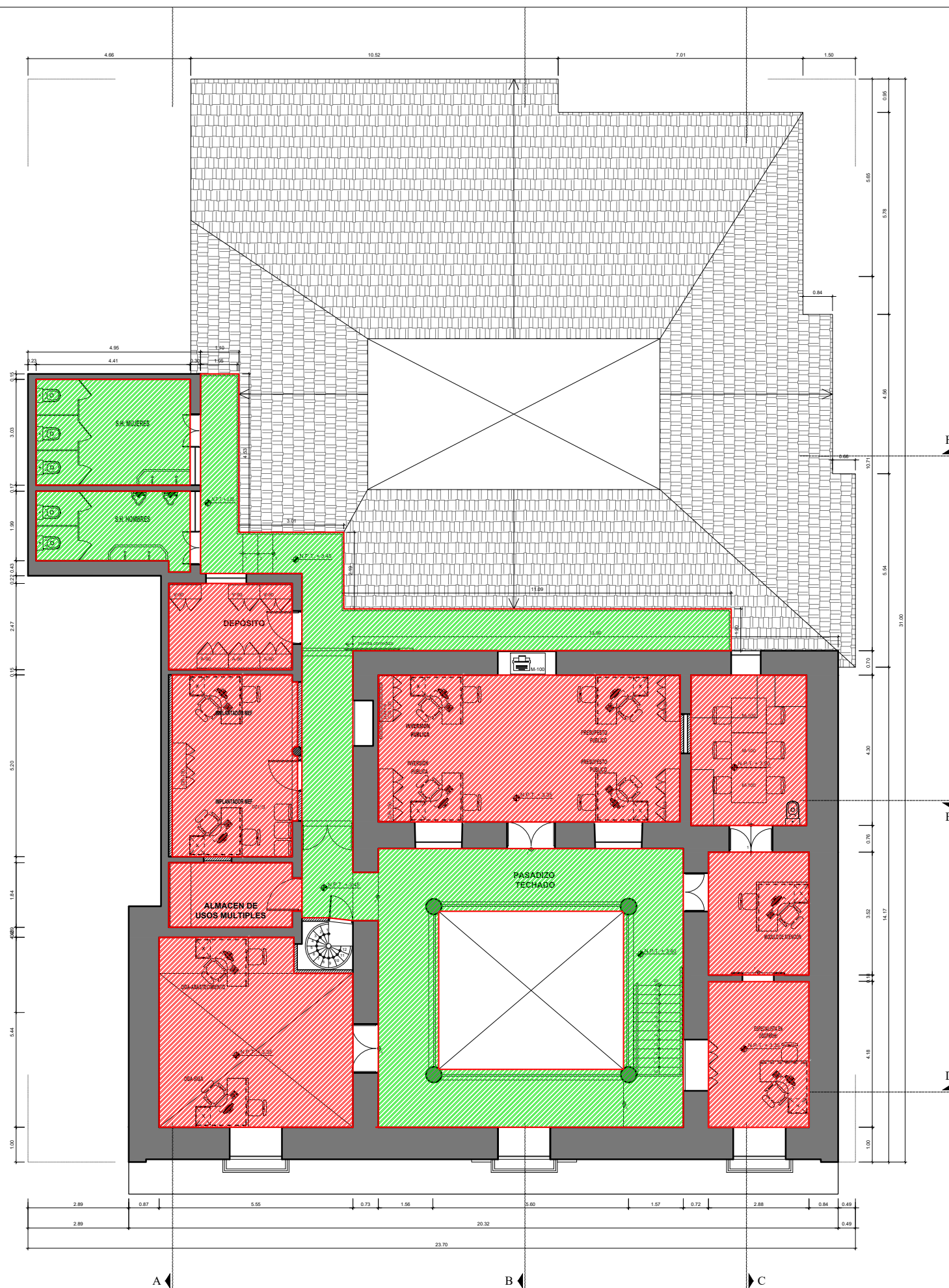
PLANO DE DISTRIBUCIÓN - 2DO PISO
