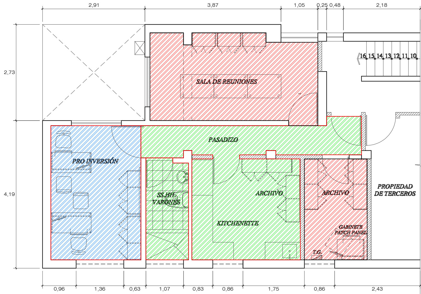
SEGUNDO PISO - ESC. 1/75
