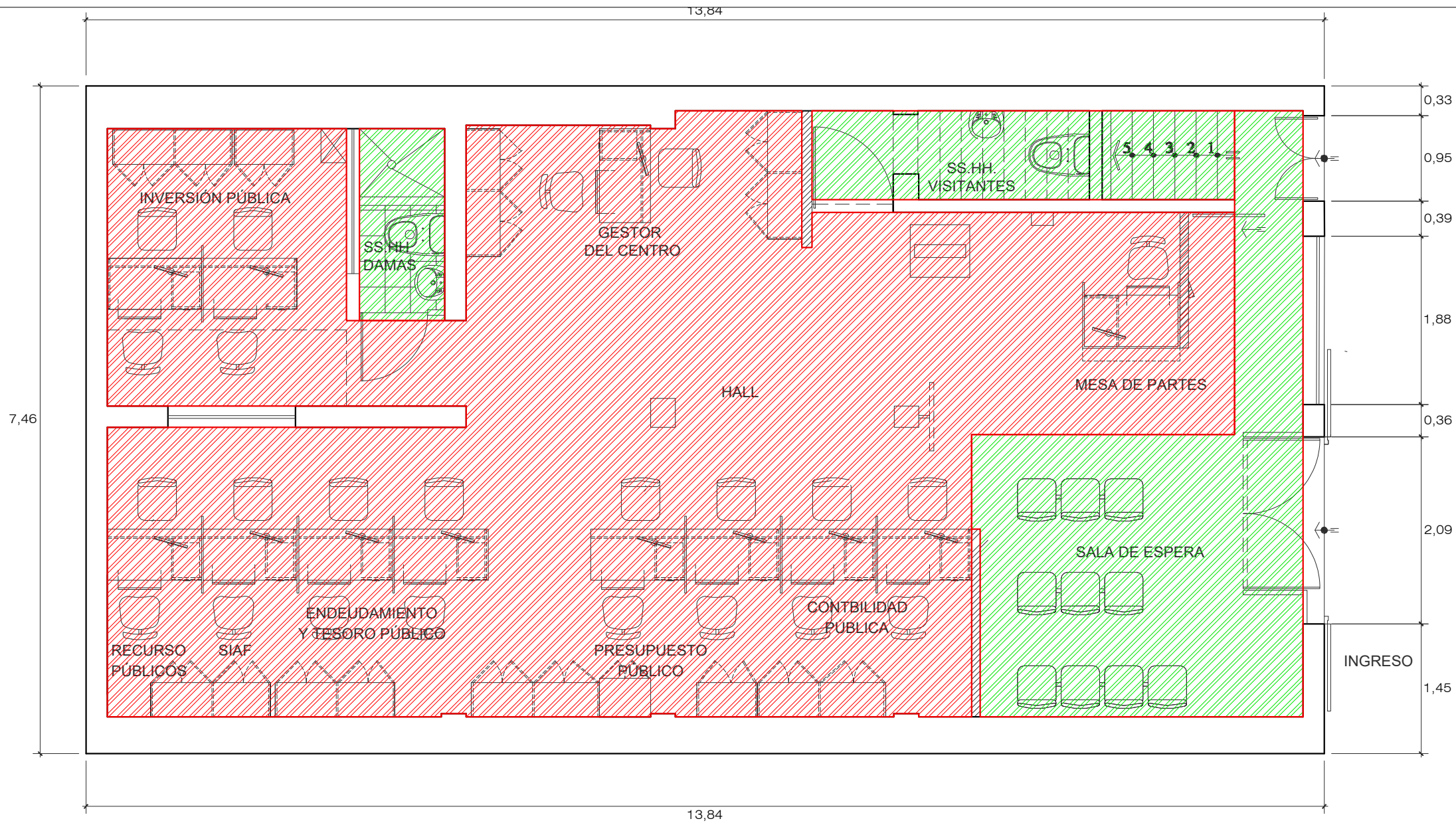
PRIMER PISO - ESC. 1/75
