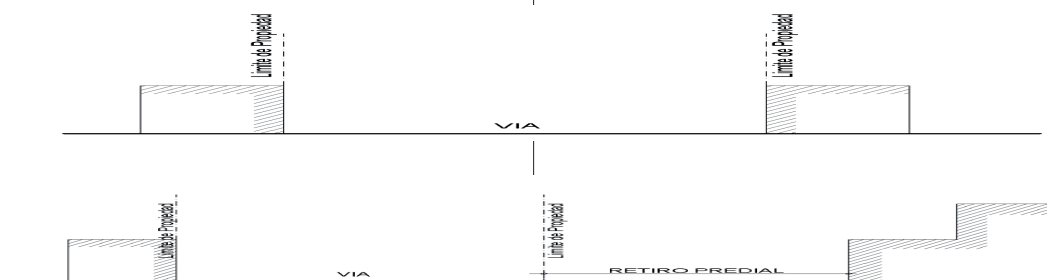
ESQUEMA DE SECCION VIAL Y RETIRO PREDIAL UNIDO A VIA Y PERFIL URBANO
