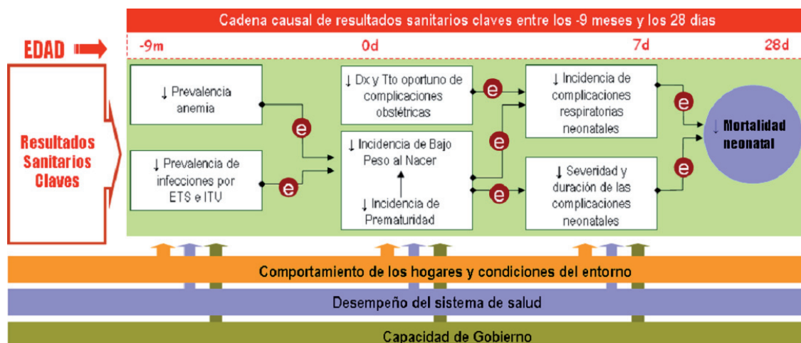
Gráfico N° 7. Principales trayectorias de causalidad asociadas a la mortalidad neonatal
