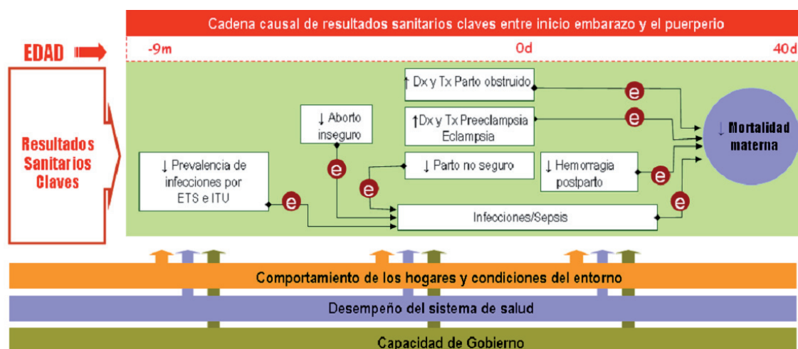
Gráfica N° 6. Principales trayectorias de causalidad asociados a la mortalidad materna
