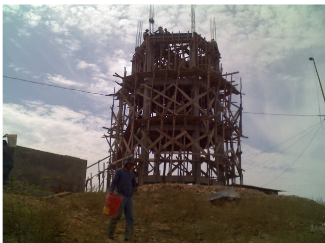
Base para la construcción del reservorio elevado
